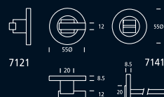
7121 - 7141 Condena - Apertura de emergencia sobre placa de 60x70mm.
