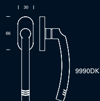
9990DK Manilla para ventana sobre placa de 66x30mm. Tornillería de fijación oculta. Handle for window on 66x30mm plate. Hidden fixing screws. Béquille de fenêtre sur plaque (66x30mm). Fixation invisible.
