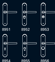
8951 Manilla sobre placa de 225x45mm. Handle on 225x45mm plate. Béquille sur plaque (225x45mm).
