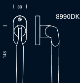
8990DK Manilla para ventana sobre placa de 66x30mm. Handle for window on 66x30mm plate. Béquille de fenêtre sur rosace ovale (66x30mm).
