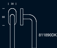
811890DK Manilla para ventana sobre placa de 66x30mm. Tornillería de fijación oculta.
