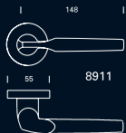
8911 Manilla sobre soporte circular de 55mm. Tornillería de fijación oculta. Handle on 55mm round support. Hidden fixing screws. Béquille sur rosace 55 mm. Fixation invisible.
