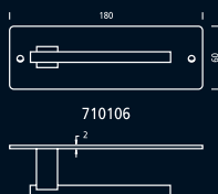
710106 Manilla sobre placa de 60 x 180 Handle on 60x180mm plate Béquille sur plaque (60x180mm)
