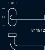
811812 Manilla para carpintería metálica o montantes reducidos sobre placa de 66x30mm. Tornillería de fijación oculta.
