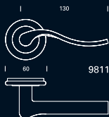
9811 Manilla sobre doble soporte circular de 60/40mm. Tornillería de fijación oculta. Handle on double 60/40mm round support. Hidden fixing screws. Béquille sur rosace de 60/40mm. Fixation invisible.
