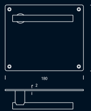
870117 Manilla sobre placa de 170x180mm. Handle on 170x180mm plate. Béquille sur plaque (170x180mm).
