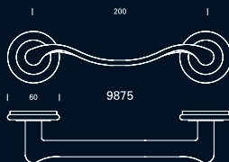
9875 Tirador de 200mm, sobre dobles soportes circulares de 60/40mm. Tornillería de fijación oculta. Pull handle, 200mm, on double 60/40mm round supports. Hidden fixing screws. Tirant de 200mm sur rosaces de 60/40mm. Fixation invisible.
