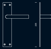
811851 Manilla sobre placa de 225x45mm. Handle on 225x45mm plate. Béquille sur plaque (225x45mm).
