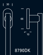
8790DK Manilla para ventana sobre placa de 66x30mm. Tornillería de fijación oculta. Handle for window on 66x30mm plate. Hidden fixing screws. Béquille de fenêtre sur rosace ovale 66x30mm. Fixation traversante invisible.
