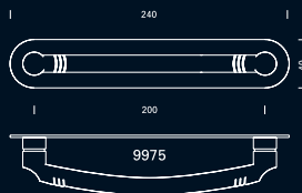
9975 Tirador de 200mm sobre placa de 240x40mm con fijación oculta. Pull handle, 200mm, on 240x40mm plate, hidden fastening. Tirant de 200mm sur plaque de 240x40mm. Fixation invisible.
