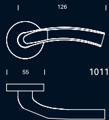
1011 Manilla sobre soporte circular de 55mm. Tornillería de fijación oculta. Handle on 55mm round support. Hidden fixing screws. Béquille sur rosace de 55mm. Fixation invisible.
