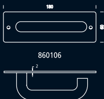
860106 Manilla sobre placa de 60 x 180 Handle on 60x180mm plate Béquille sur plaque (60x180mm)
