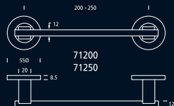
71200 - 71250 Tirador de 200 y 250mm sobre soportes circulares de 55mm.
