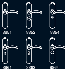
8851 Manilla sobre placa de 245x50mm. Tornillería de fijación oculta. Handle on 245x50mm plate. Hidden fixing screws. Béquille sur plaque (245x50mm). Fixation invisible.
