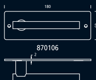
870106 Manilla sobre placa de 60 x 180 Handle on 60x180mm plate Béquille sur plaque (60x180mm)
