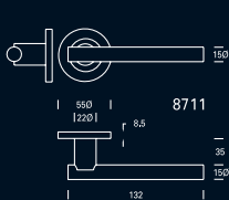
8711 Manilla sobre soporte circular de 55mm. Tornillería de fijación oculta. Handle on 55mm round support. Hidden fixing screws. Béquille sur rosace ø55 mm. Fixation traversante invisible.
