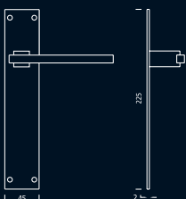
7151C Manilla sobre placa de 225x45mm. Handle on 225x45mm plate. Béquille sur plaque (225x45mm).
