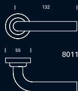
8011 Manilla sobre soporte circular de 55mm. Tornillería de fijación oculta. Handle on 55mm round support. Hidden fixing screws. Béquille sur rosace de 55mm. Fixation invisible.
