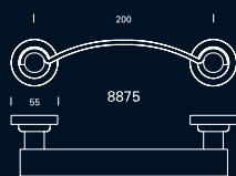
8875 Tirador de 200mm, sobre soportes circulares de 55mm. Tornillería de fijación oculta. Pull handle, 200mm, on 55mm round supports. Hidden fixing screws. Tirant, 200mm, rosace de 55mm. Fixation invisible.
