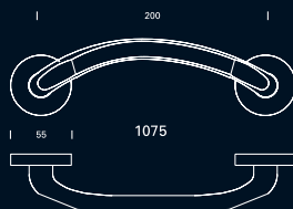
1075 Tirador de 200mm sobre soportes circulares de 55mm. Tornillería de fijación oculta. Pull handle, 200mm, on 55mm round supports. Hidden fixing screws. Tirant, 200mm sur rosaces de 55mm. Fixation invisible.
