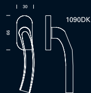
1090DK Manilla para ventana sobre placa de 66x30mm. Tornillería de fijación oculta. Handle for window on 66x30mm plate. Hidden fixing screws. Béquille de fenêtre sur plaque (66x30mm). Fixation invisible.
