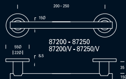
87200 - 87250 Tirador de 200 y 250mm sobre soportes circulares de 55mm. Tornillería de fijación oculta. Pull handle, 200 and 250mm, on 55mm round supports. Hidden fixing screws.
