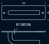
81180106 Manilla sobre placa de 60 x 180 Handle on 60x180mm plate Béquille sur plaque (60x180mm)
