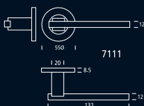
7111 Manilla sobre soporte circular de 55mm.
