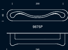
9875P Tirador de 200mm, sobre placa de 240x40mm con fijación oculta. Pull handle, 200mm, on 240x40mm plate, hidden fastening. Tirant, 200mm sur plaque (240x40mm). Fixation invisible.
