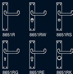
8651R Manilla sobre placa de 225x45mm. Handle on 225x45mm plate. Béquille sur plaque (225x45mm).
