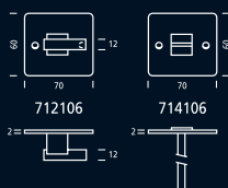
712106 - 714106 Condena - Apertura de emergencia sobre placa de 60x70mm.
