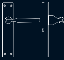
8951 Manilla sobre placa de 225x45mm. Handle on 225x45mm plate. Béquille sur plaque (225x45mm).
