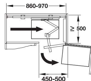
3. Extraído y girado hacia la derecha
